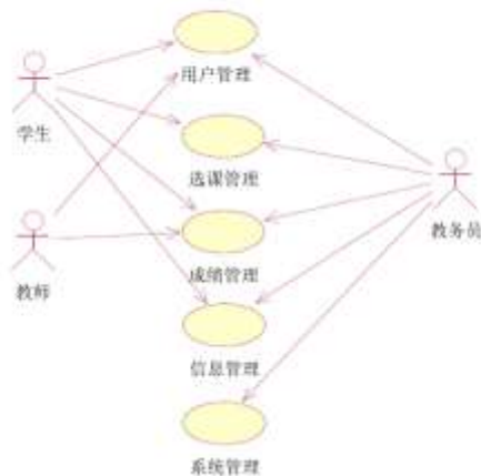
系统用例图
