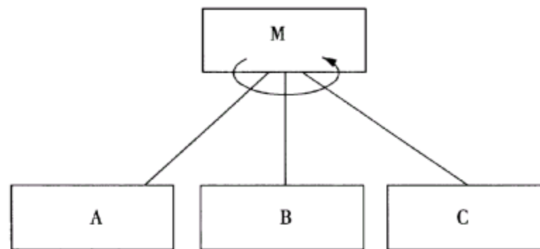
循环调用
