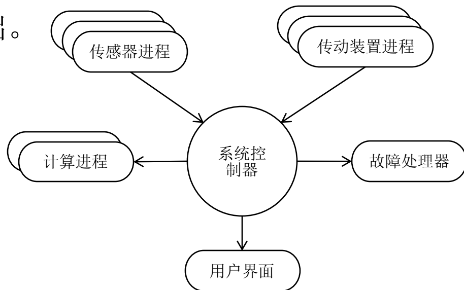
管理者模型
